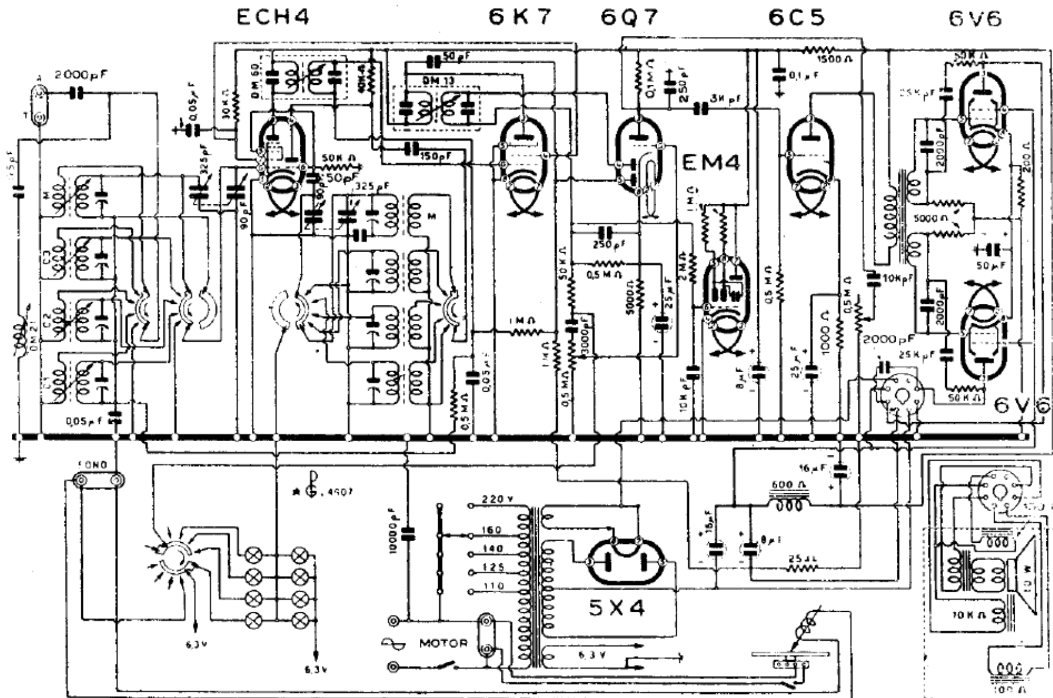
Lo schema elettrico del radiofonografo mod. 745 RF
